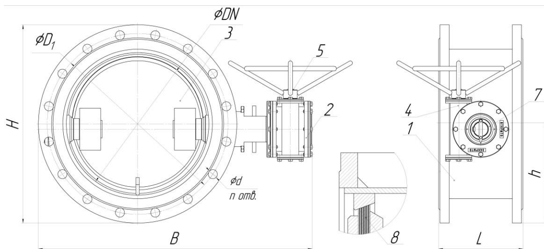
Габаритный чертёж
