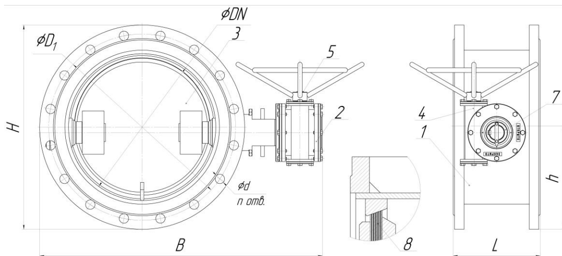
Габаритный чертеж
