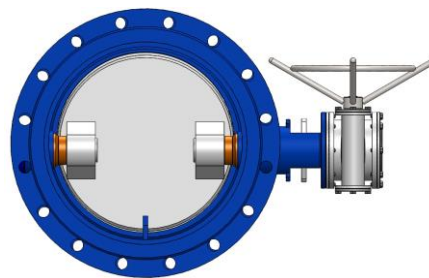
Вид сзади
