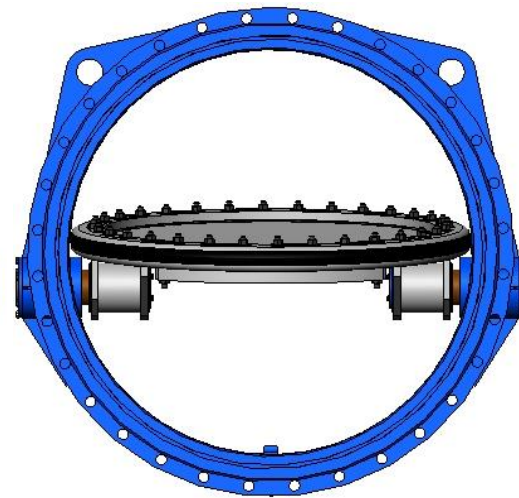
Положение «Открито»
